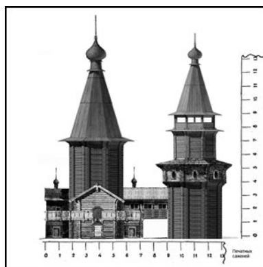
Рис.3. Западный фасад Воскресенской церкви (реконструкция).
