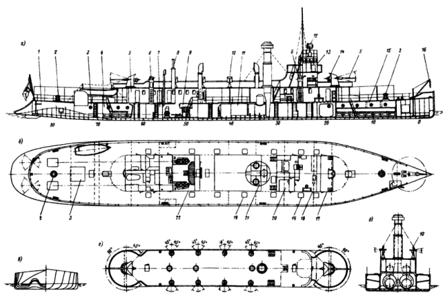
Чертёж небронированной канонерской лодки типа «Бурят», к которому относился «Орочанин»
